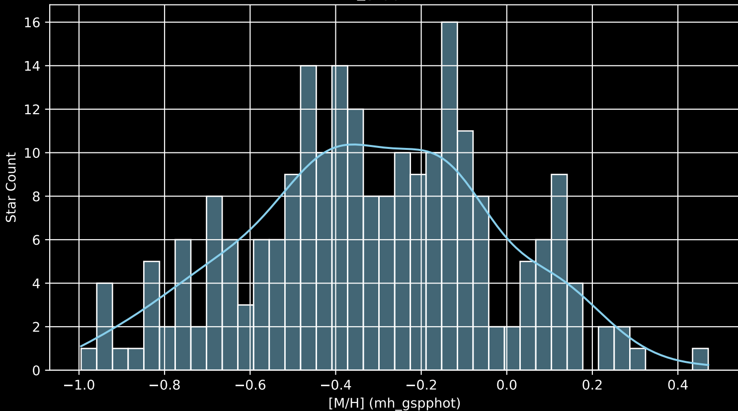
GALAH DR4 Field: [7201] [M/H] (mh_gspphot) (n= 224)
