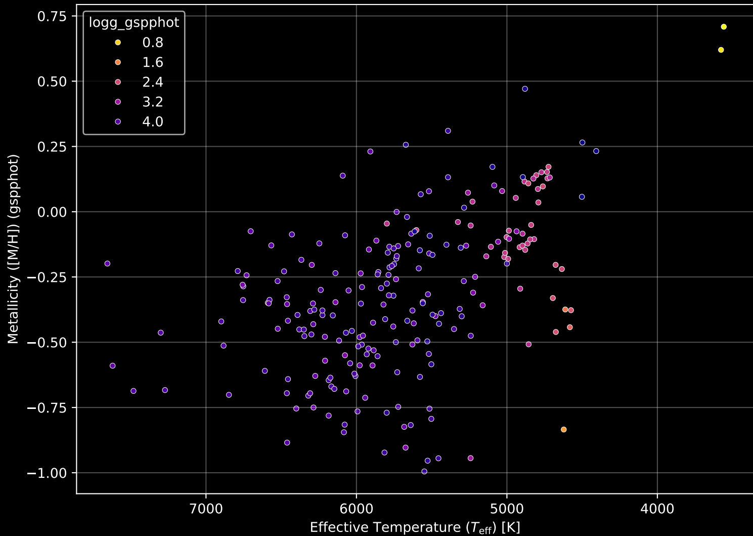
GALAH DR4 Field: [7201] Stellar Population Parameters (n= 226)
